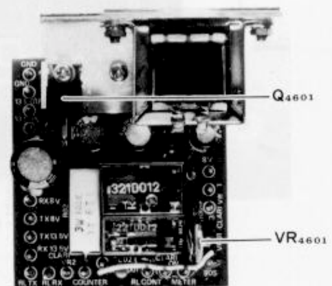
AVR UNIT
